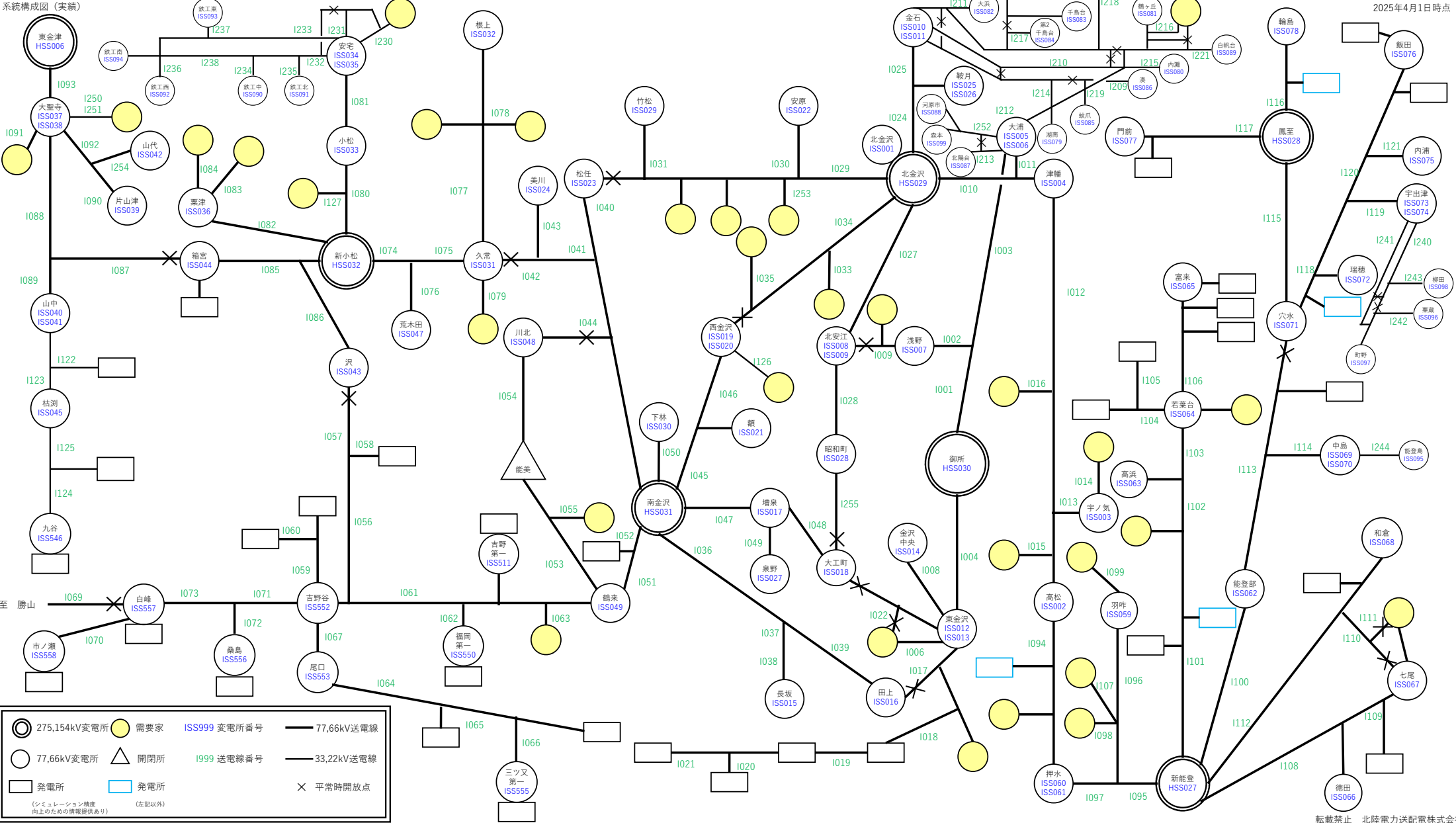
系統構成図（実績）
