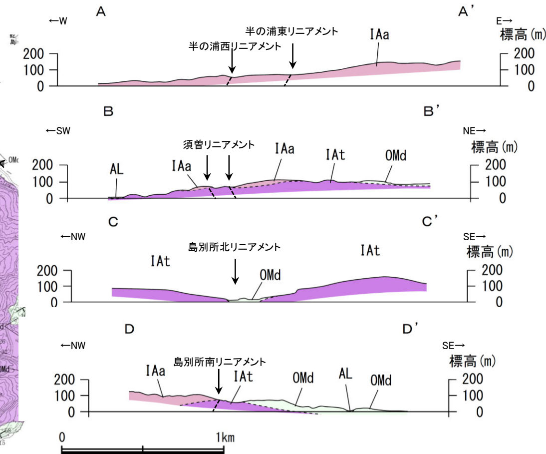
地質断面図
