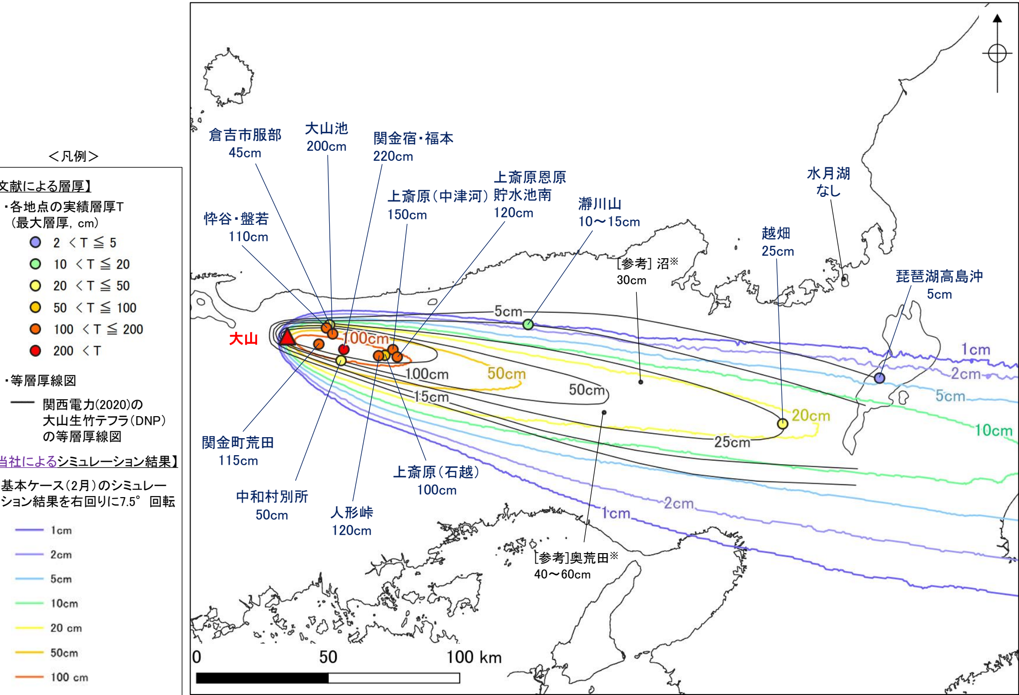
大山生竹テフラの当社シミュレーション結果と文献(関西電力(2020))による層厚の比較
