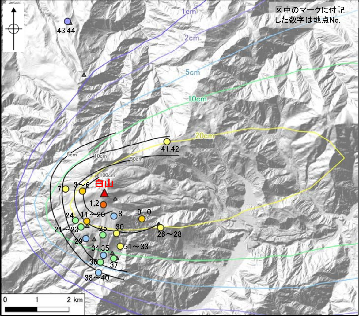
南竜火山灰層のシミュレーション結果と 文献による層厚の比較
