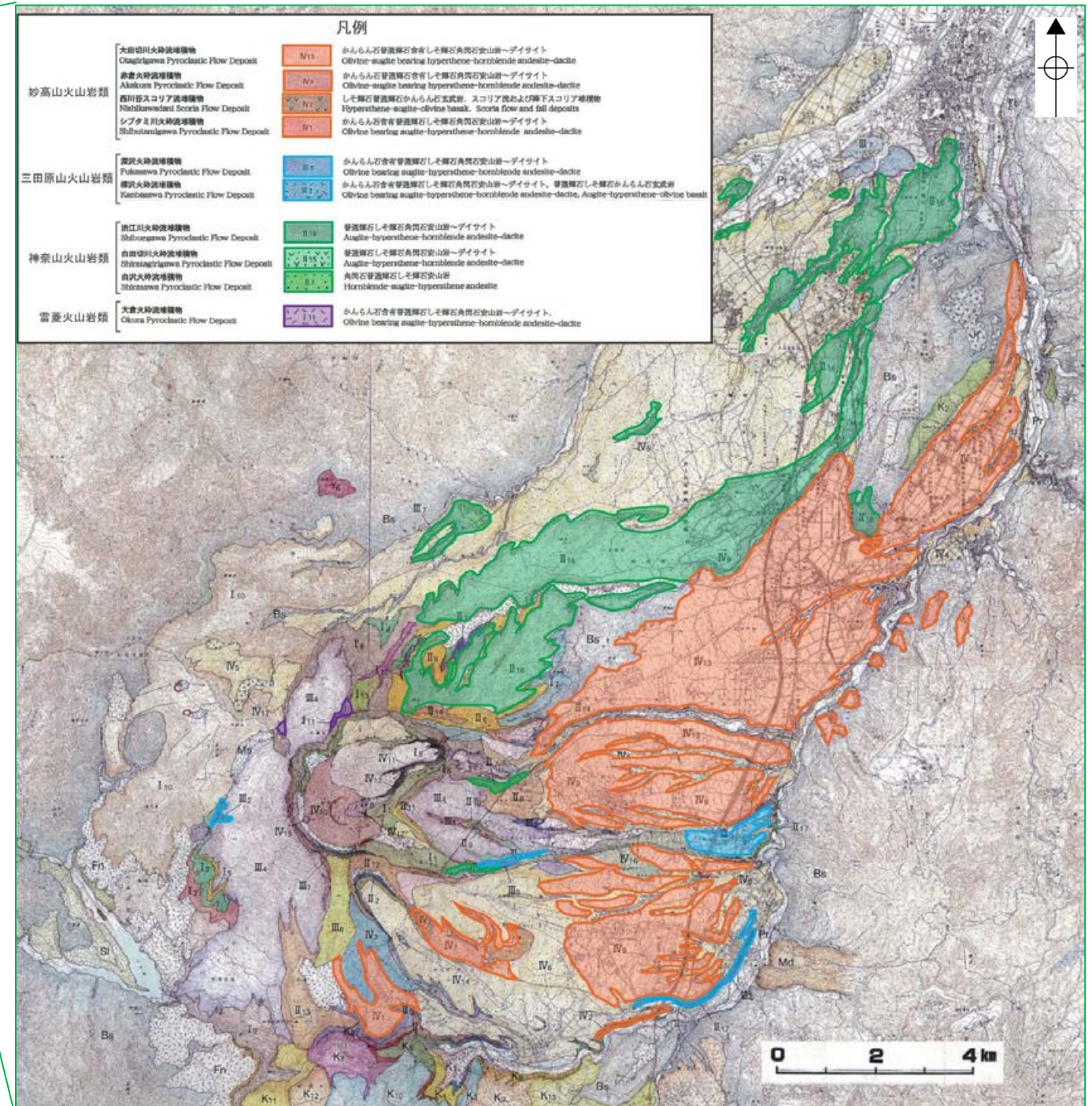
妙高山の地質図 (早津(2008)に一部加筆)
