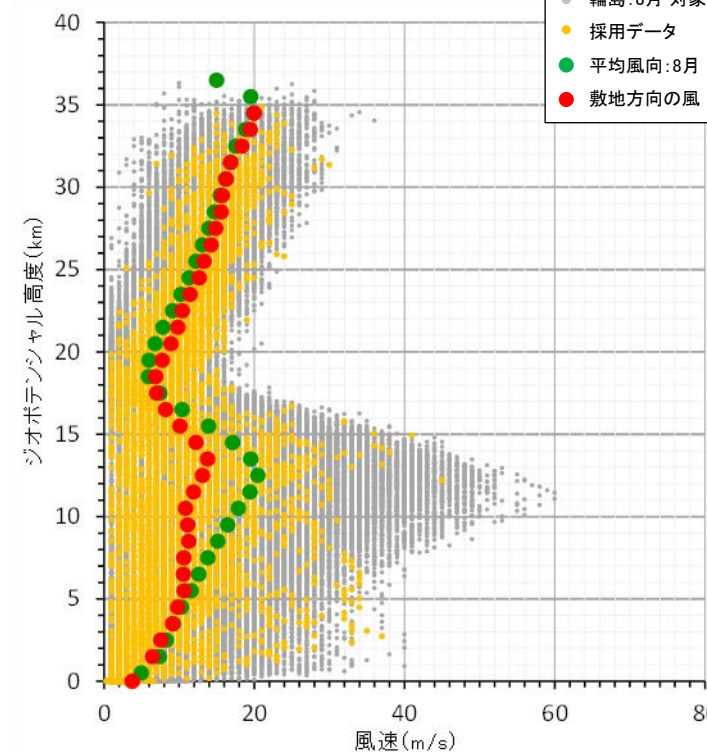
解析に用いる風データ
