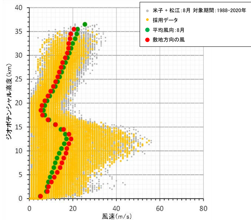
解析に用いる風データ
