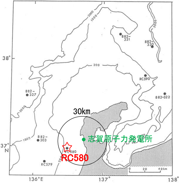
調査位置図 (町田(1989)に一部加筆)
