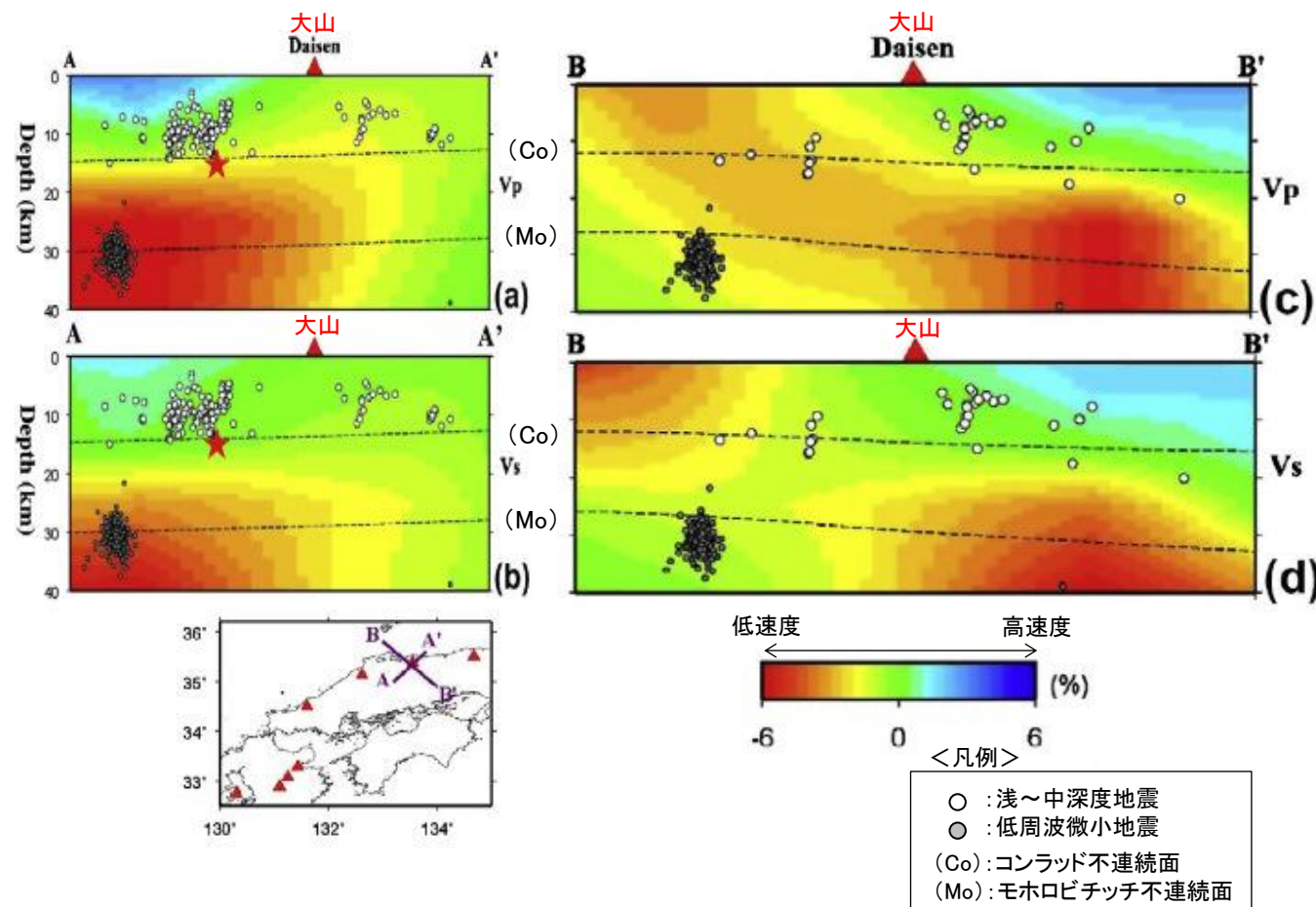
大山周辺の地震波速度構造 (Zhao et al.(2011)に一部加筆)
