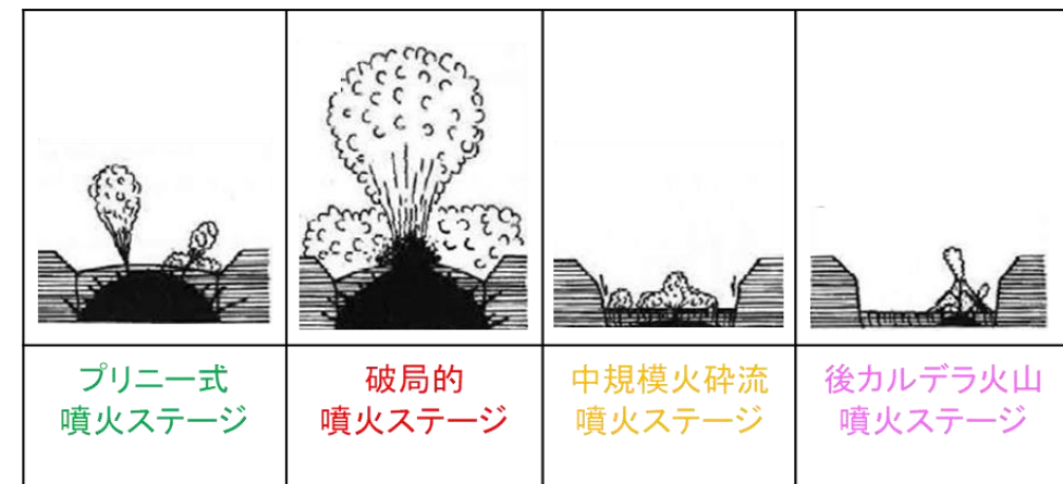
噴火ステージ区分 (Nagaoka(1988)に基づき作成)
