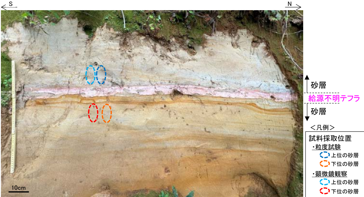
余地地点の露頭の拡大写真
