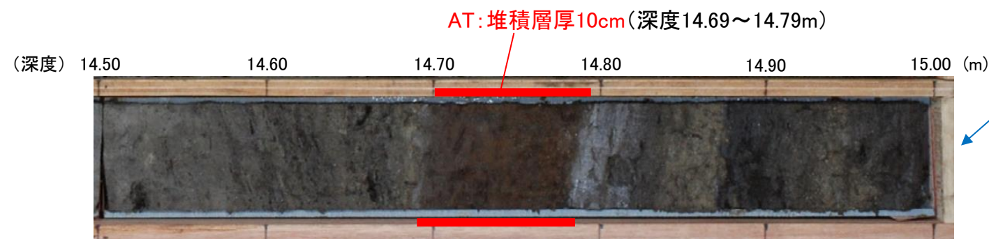
コア写真
