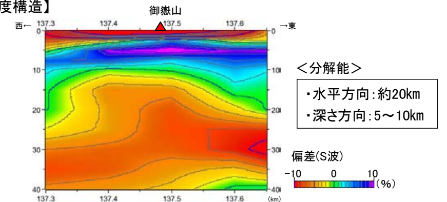
御嶽山の山頂を通る東西方向のS波鉛直断面 (Matsubara et al.(2022)に基づき作成)
