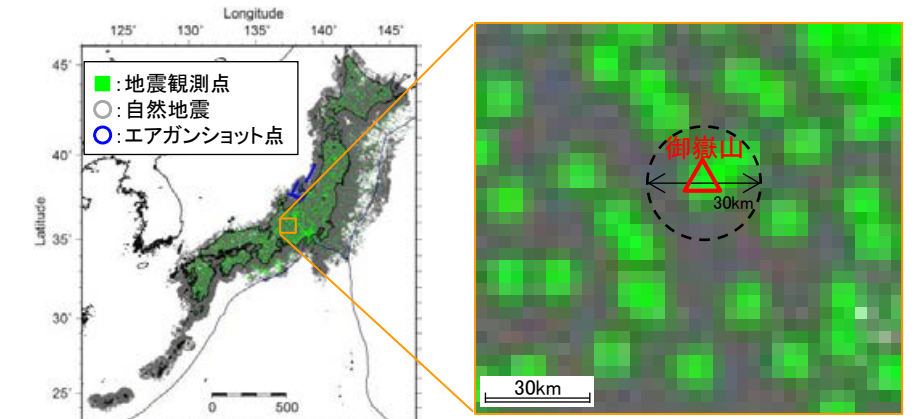
検討に用いる地震計の配置状況 (Matsubara et al.(2022)に一部加筆)
