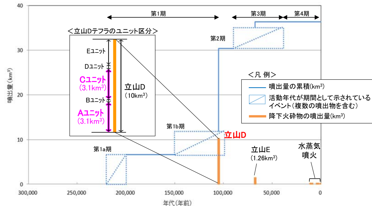
立山の階段ダイヤグラム
