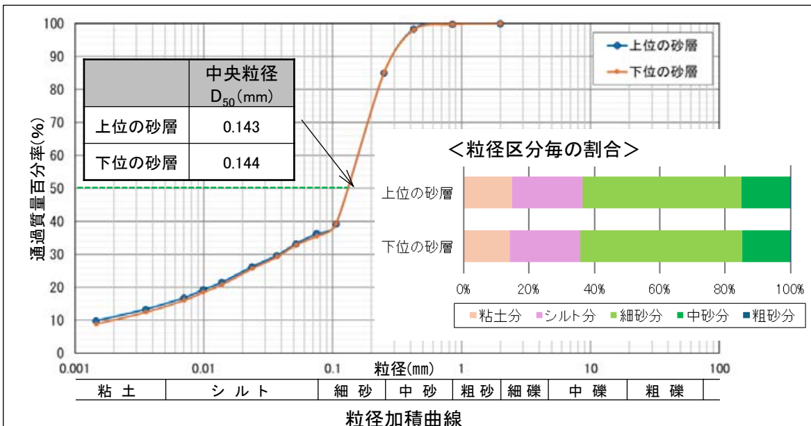
【粒径(粒度試験結果)】 試料採取位置 2024年10月撮影 試料採取2024年10月
