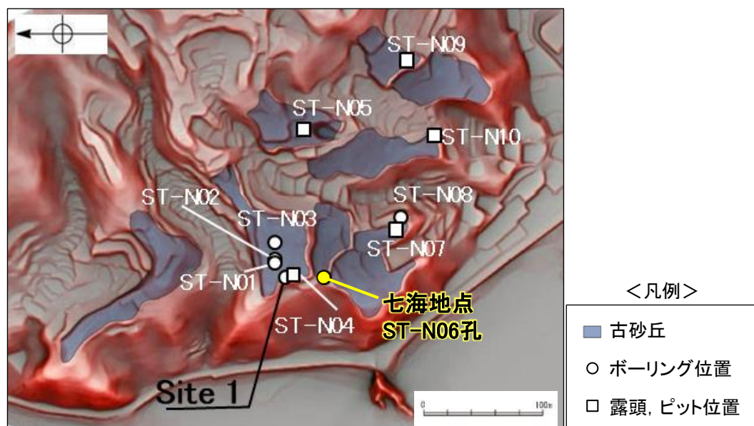
地形面区分图
