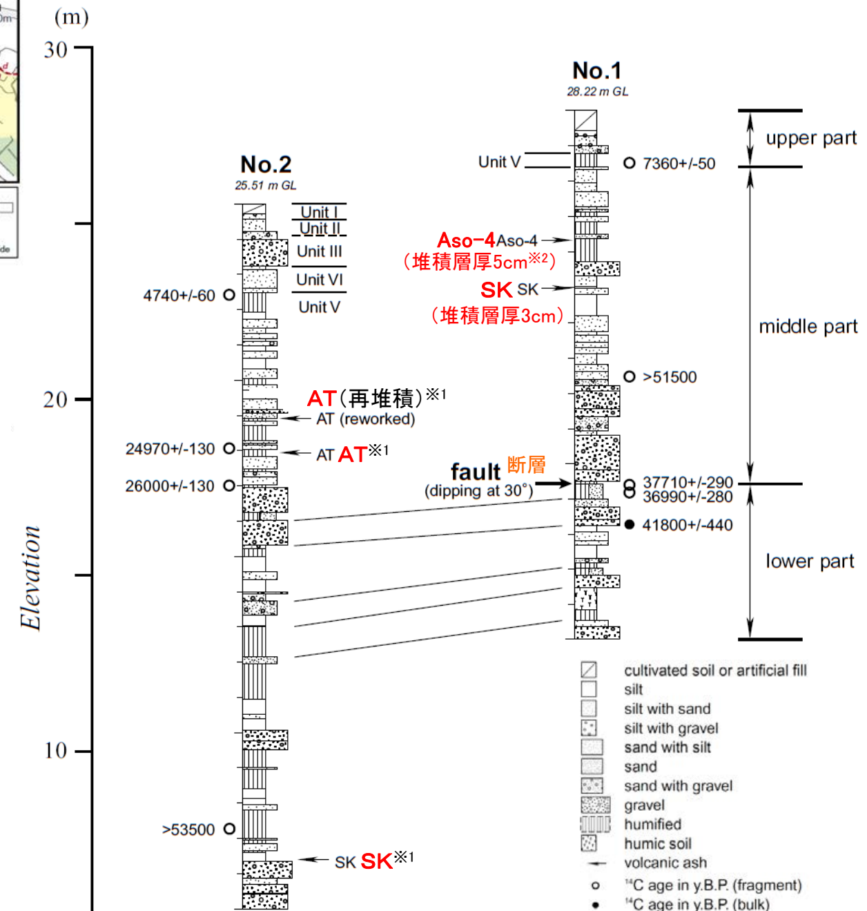
水白地点のボーリング調査位置 (杉戸ほか(2004)に一部加筆)
