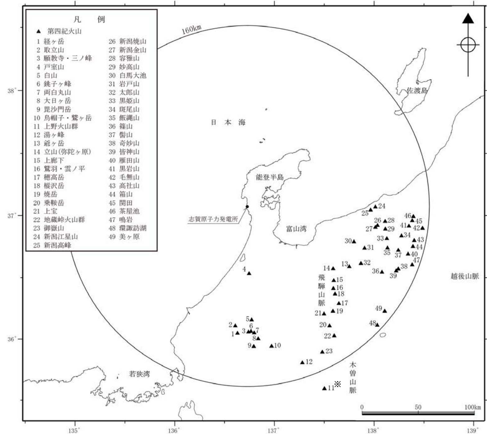
地理的領域内の第四紀火山の位置
