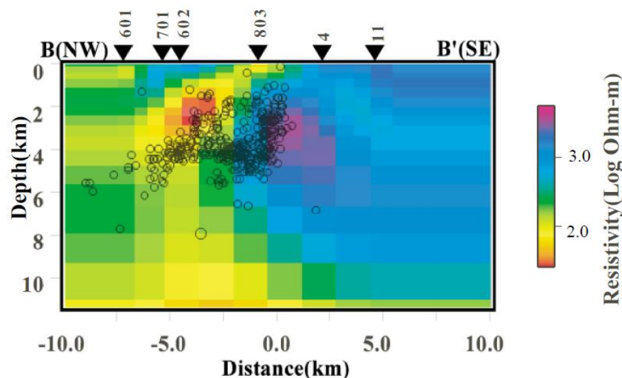
2測線の比抵抗構造二次元断面 (Kasaya et al., 2002)
