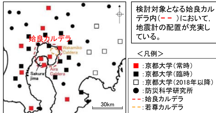
検討に用いる地震計の配置状況 (為栗ほか(2022)に一部加筆)
