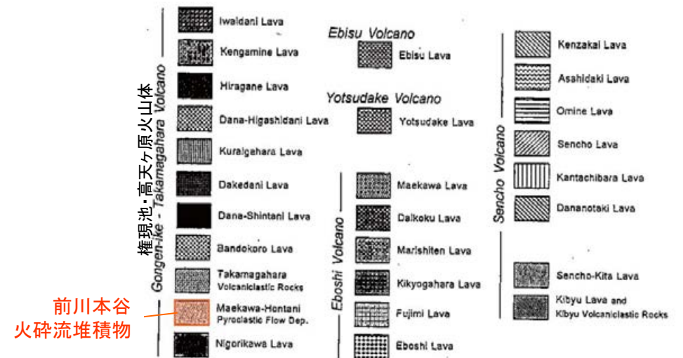
乗鞍岳の地質図 (中野(1998)に一部加筆)
