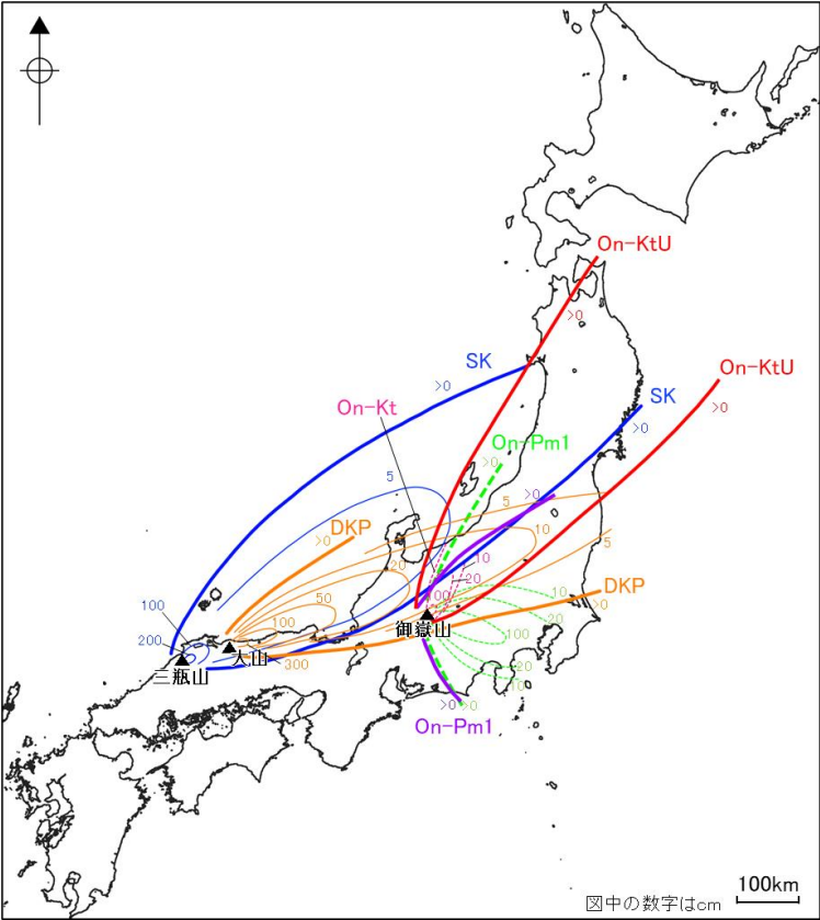
御嶽湯町テフラ及び国内の主なVEI6クラスの広域テフラの分布 (Matsu’ura and Komatsubara(2024), 町田・新井(2011)に示された等層厚線に基づき作成)
