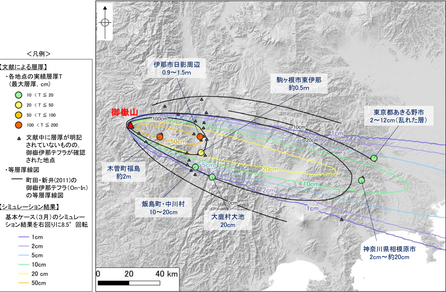
御嶽伊那テフラのシミュレーション結果と文献による層厚の比較
