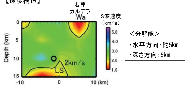
始良カルデラの中央部を通る東西方向のS波鉛直断面 (為栗ほか(2022)に一部加筆)
