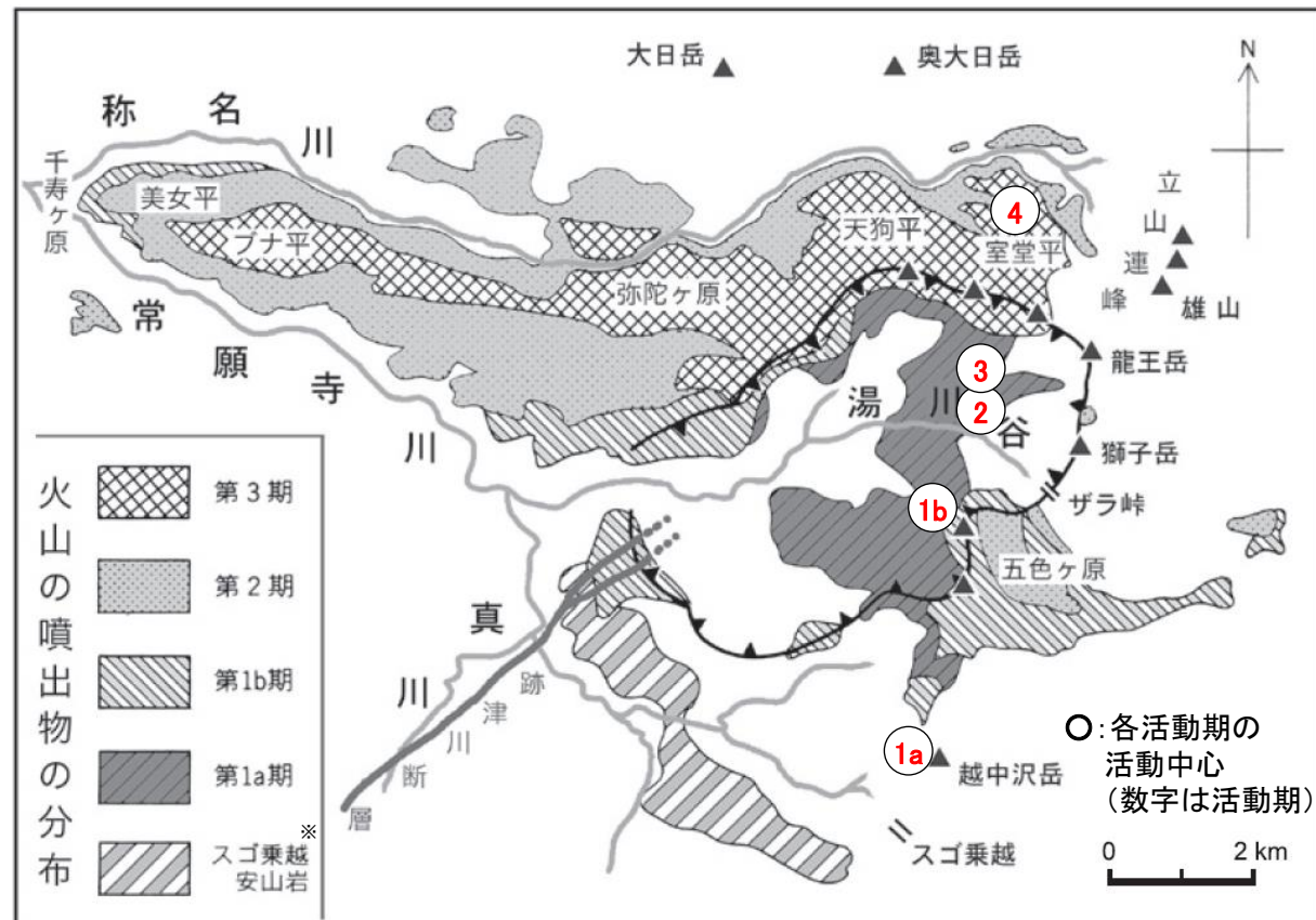
立山の地質図
