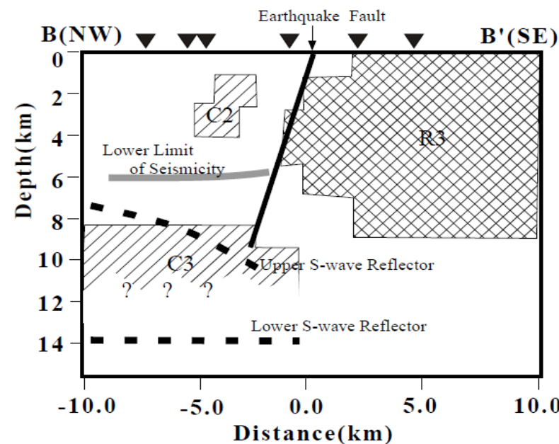
単純化した二次元比抵抗構造 (Kasaya et al., 2002)
