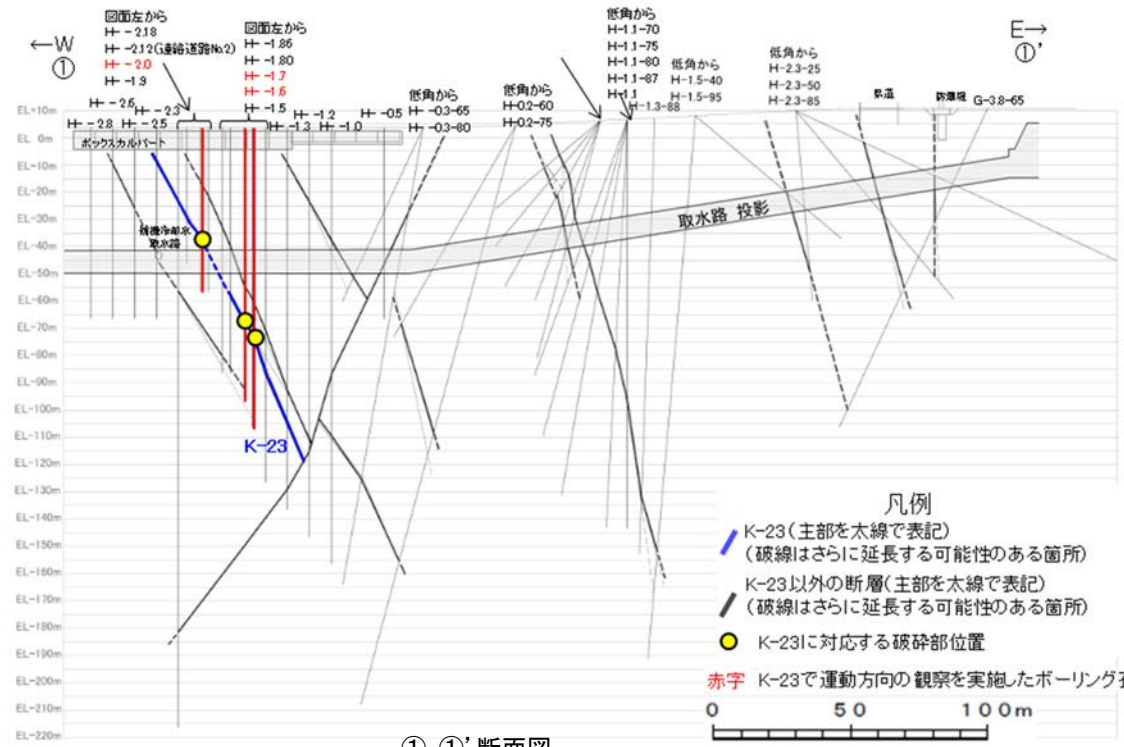
①-①' 断面図
