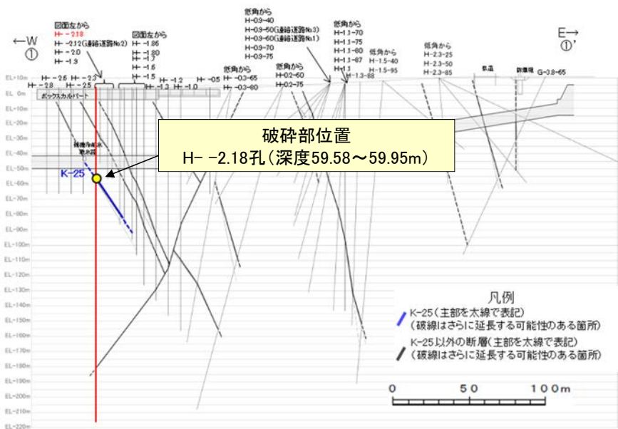
①-①' 断面図
