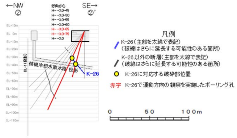
②-②' 断面図
