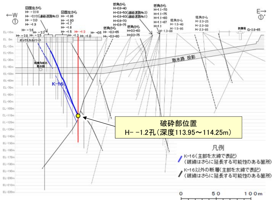
①-①'断面図
