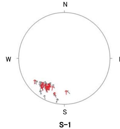
I・右系 (走向: I系, 横ずれ卓越の右横ずれ断層)
