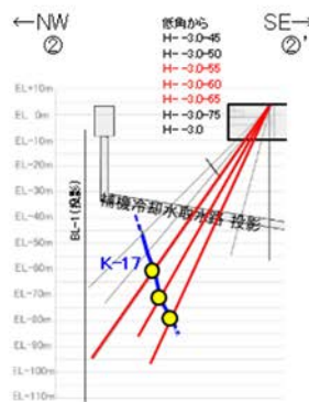
②-②' 断面図
