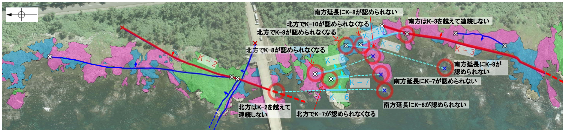
海岸部露岩域の断層の分布図
