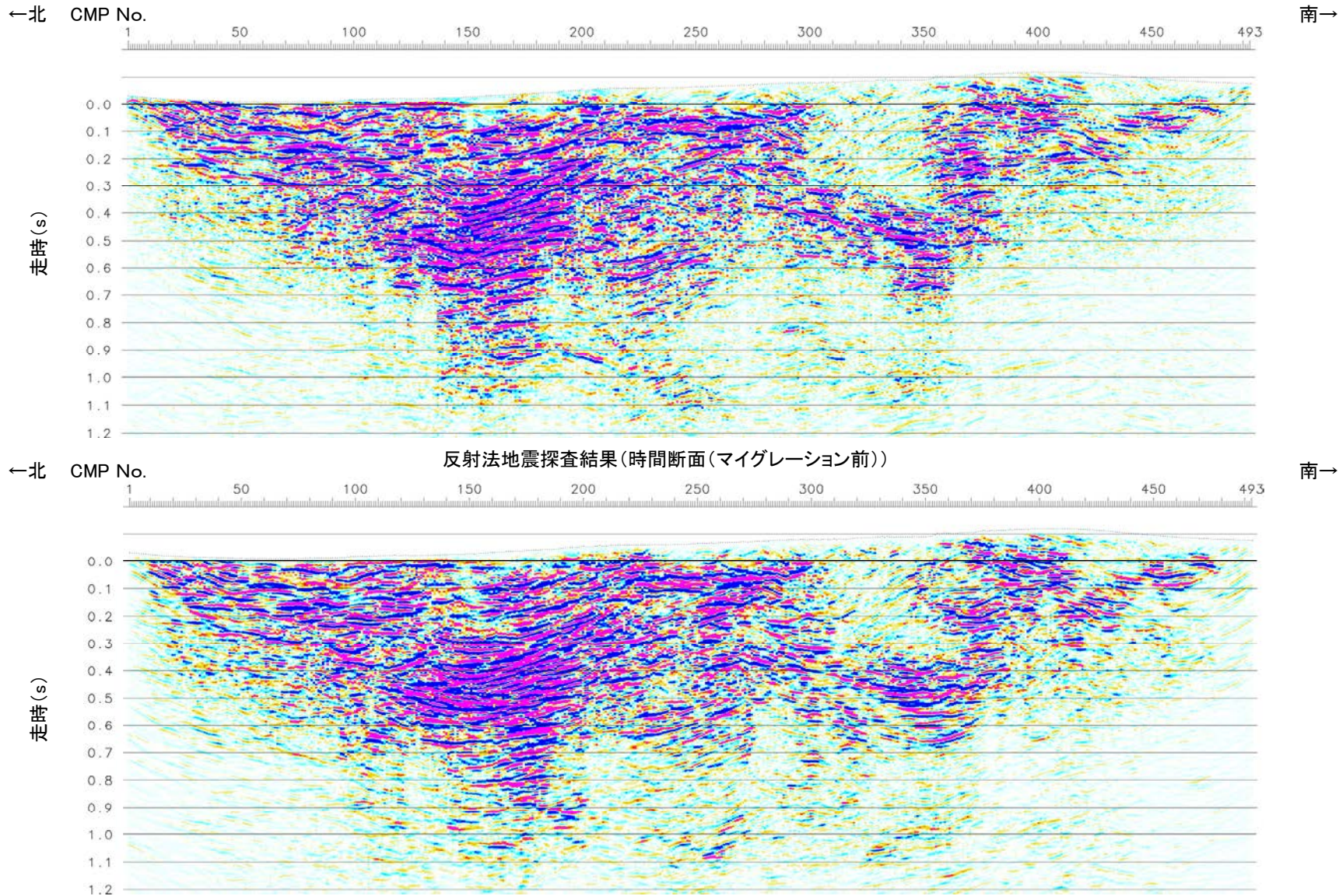
【時間断面(マイグレーション前，後)(小林ほか，2020)】
