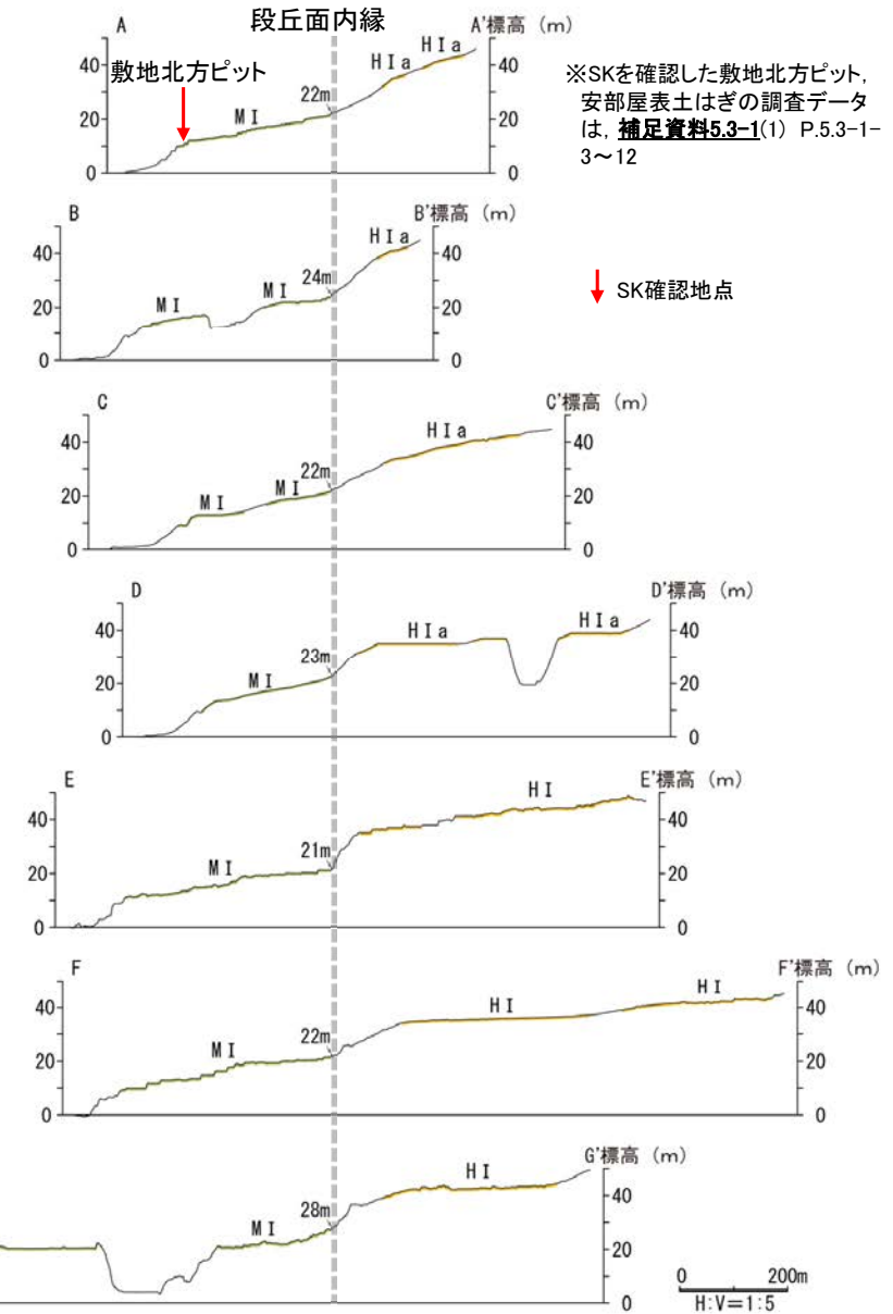
地形断面図
