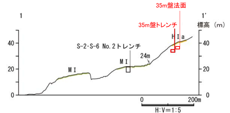
地形断面図
