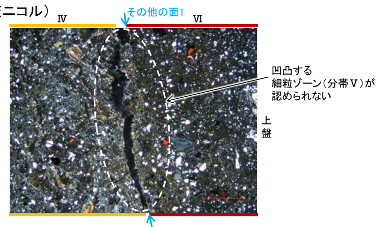
(直交ニコル)
