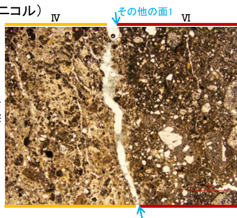
(単ニコル)
