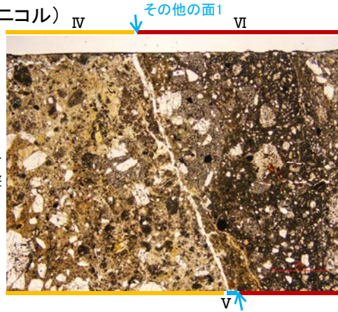
(直交ニコル)
