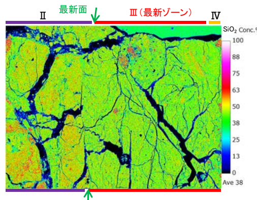
SiO 2
