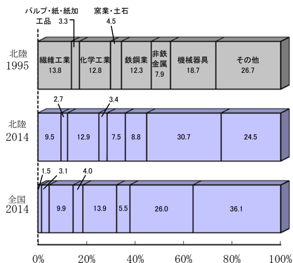
大口使用電力量の産業別構成比
