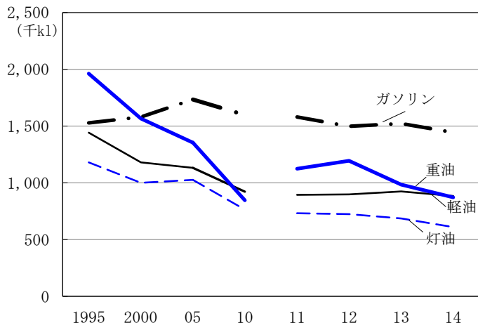
燃料油製品別販売量の推移(北陸)
