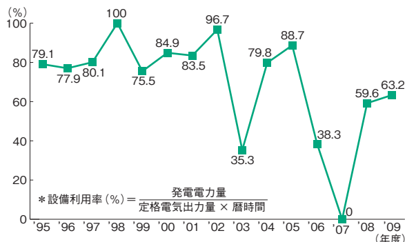
■志賀原子力発電所 設備利用率の推移
