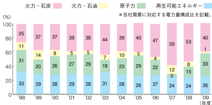
■発電電力量構成比率の推移
