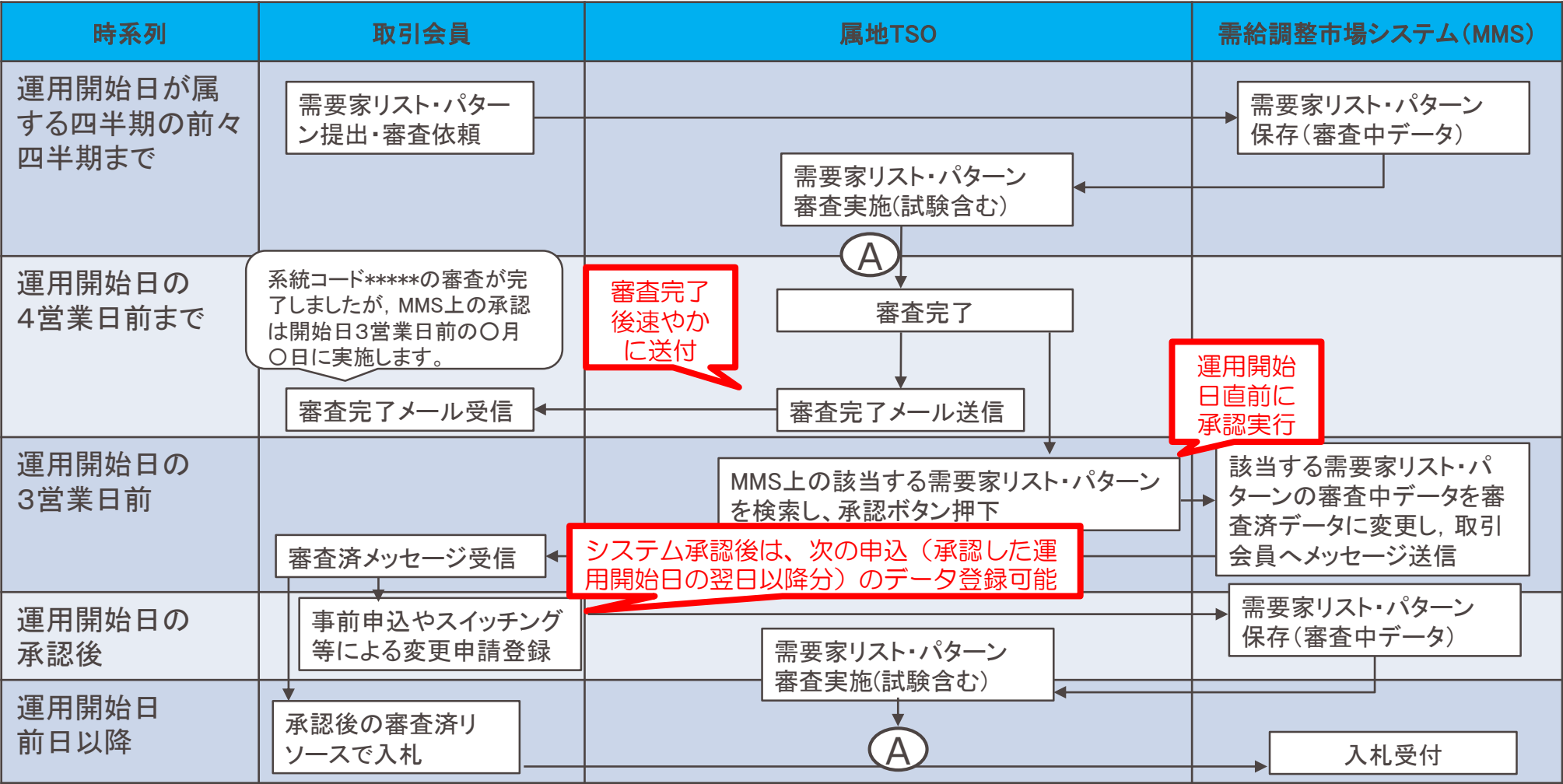
【需要家リスト・パターン変更時の業務フロー】
