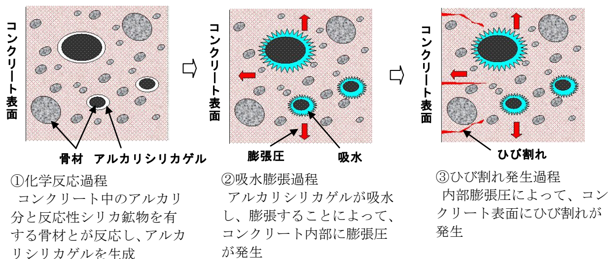
図1-5 アルカリシリカ反応のメカニズム
