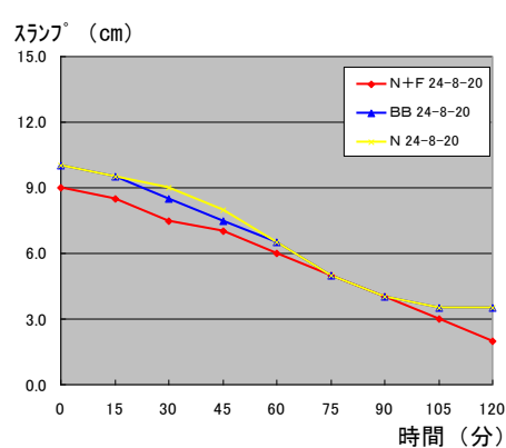
図5-5 南条産骨材のスランプロス
